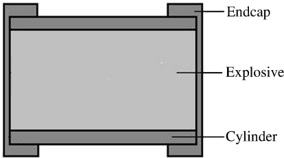
图 1 烤燃弹试样结构简图
