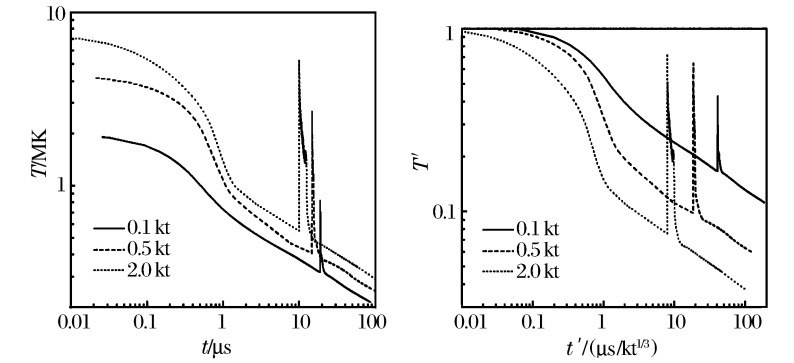
图 4 不同当量的火球中心温度和归一化火球中心温度 Fig. 4 Temperature and scaled temperature at fireball center for different yields
