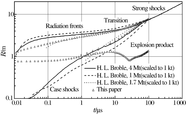
图 1 1 kt 当量火球阵面计算结果
