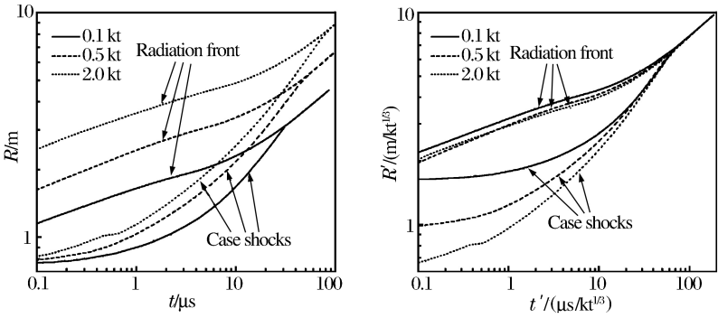
图 2 不同当量的火球阵面 Fig. 2 Fireball fronts for different yields
