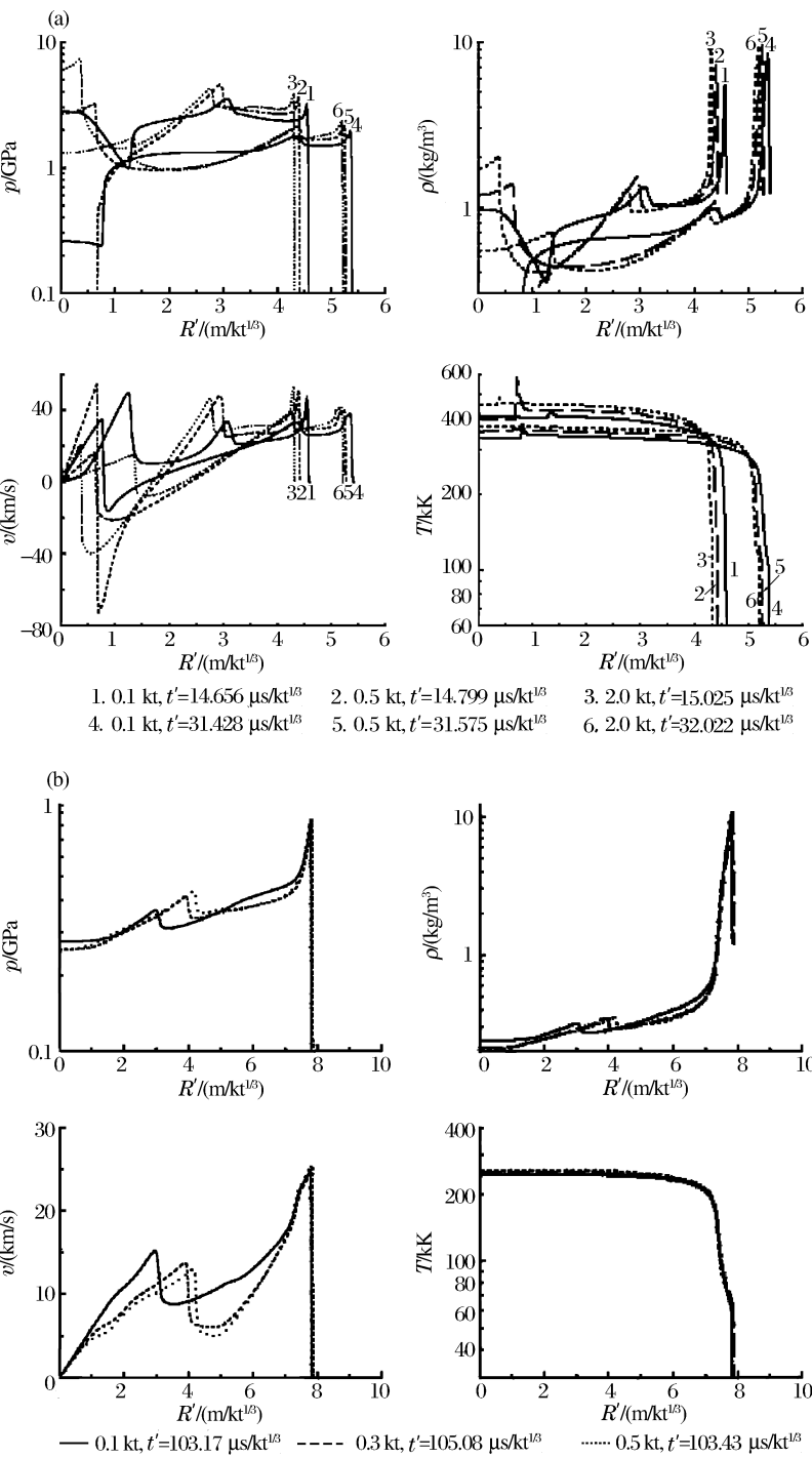
图 5 不同比例时间、不同当量的物理参量
