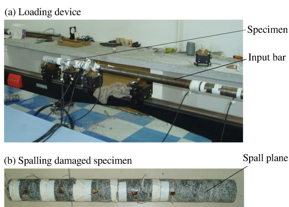
图 2 花岗岩试样层裂实验
