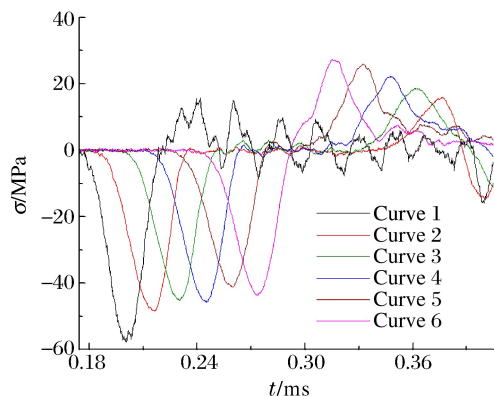
图 3 试样中的透射波
