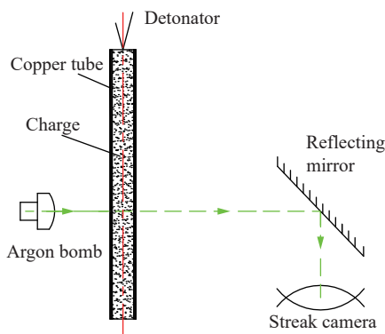
图 2 狭缝扫描试验布局图
