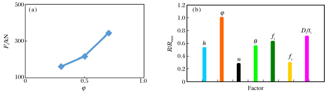
图 7 各因素对冲击力平台值的影响
