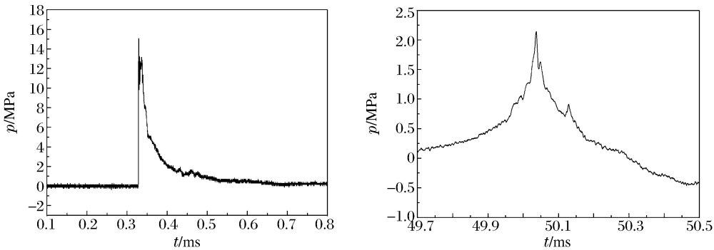
图 10 距离 3 号药柱 0.7\text{ m} 处冲击波压力与气泡第一次脉动压力时程曲线
