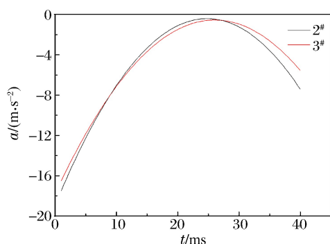
图 13 脉动过程中气泡膨胀、收缩加速度随时间的变化
