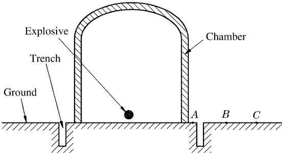
图 1 塔体结构示意图 Fig.1 Schematic of the chamber
