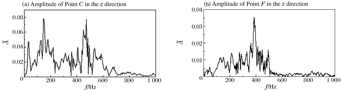
图 7 垂直方向振动的频谱分析
