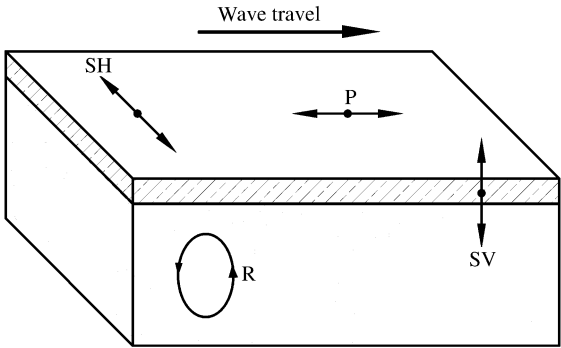
图 6 介质中的地震波
