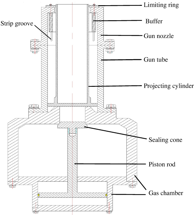
图 3 水冲击实验装置结构
