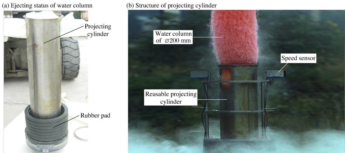
图 6 惯性抛射装置的水柱发射实验 Fig. 6 Photo of device for ejecting water column
