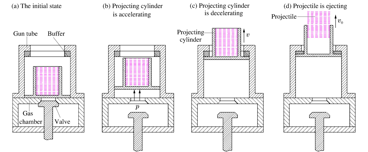
图 1 基于气体炮加载技术的惯性抛射原理示意图
