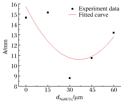
图 8 不同工况下铝粉火焰预热区厚度
