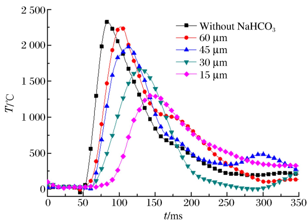
图 6 不同工况下铝粉火焰温度变化
