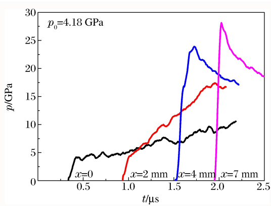
图 2 CL-20 混合炸药在距冲击波入射面不同距离处的内部压力-时间曲线
