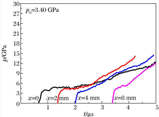
图 4 CL-20/FOX-7 混合炸药在距冲击波入射面不同距离处的内部压力-时间曲线
