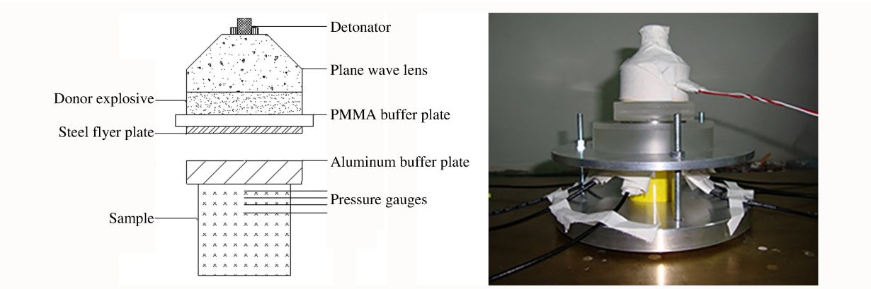
图 1 炸药驱动飞片冲击起爆实验装置示意图及照片 Fig.1 Diagram and photo of shock initiation experimental apparatus
