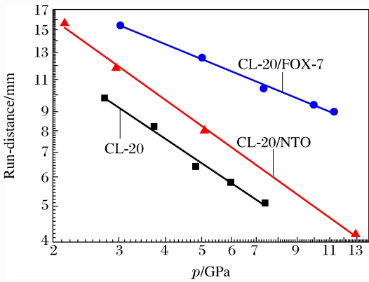
图 8 三种炸药的 POP 关系图 Fig. 8 Pop plots for the three explosives
