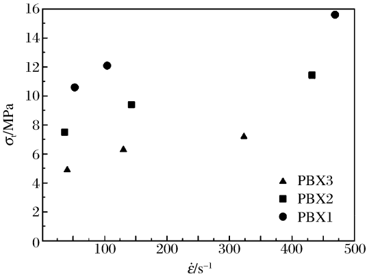
图 7 3 种 PBX 炸药试样不同应变率下的拉伸强度
