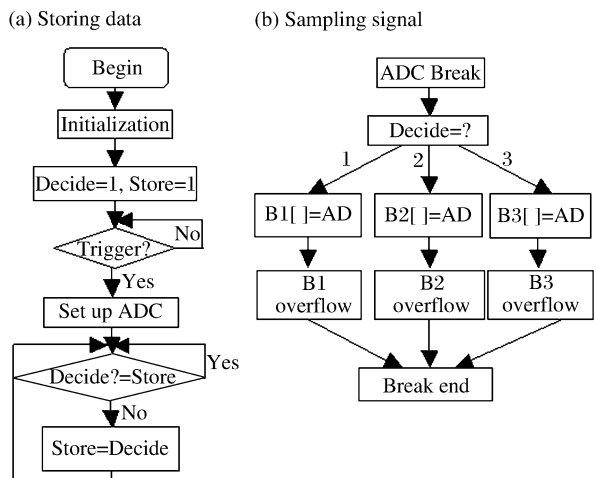
图 2 信号采集存储程序流程图
