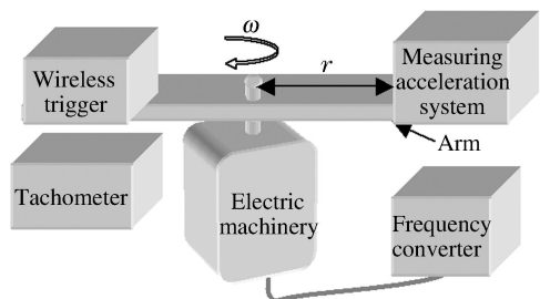
图 3 加速度静态标定实验示意图
