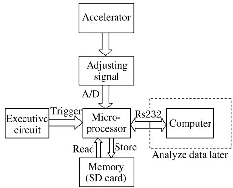
图 1 小型加速度测量系统的硬件构成
