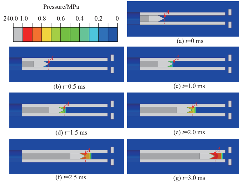
图 2 炮弹前平面激波的动态演化过程
