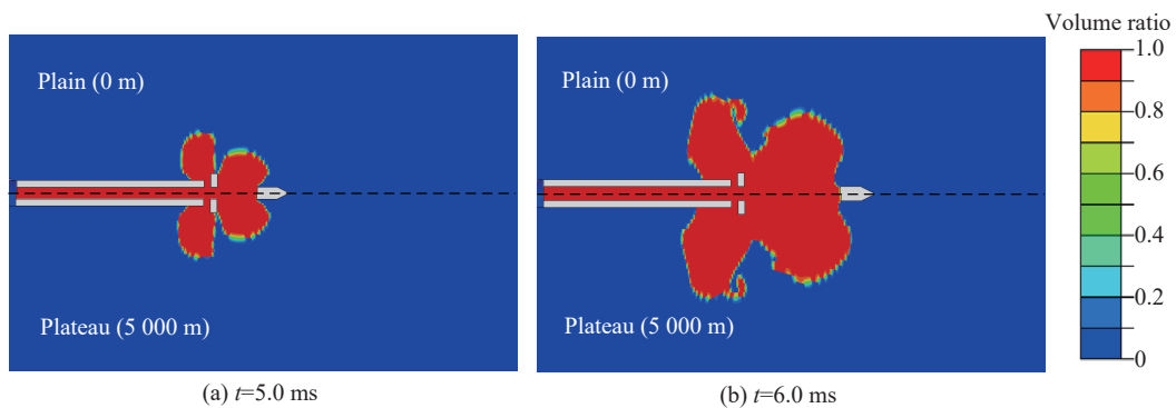
图 9 平原与高原环境下火药燃气分布
