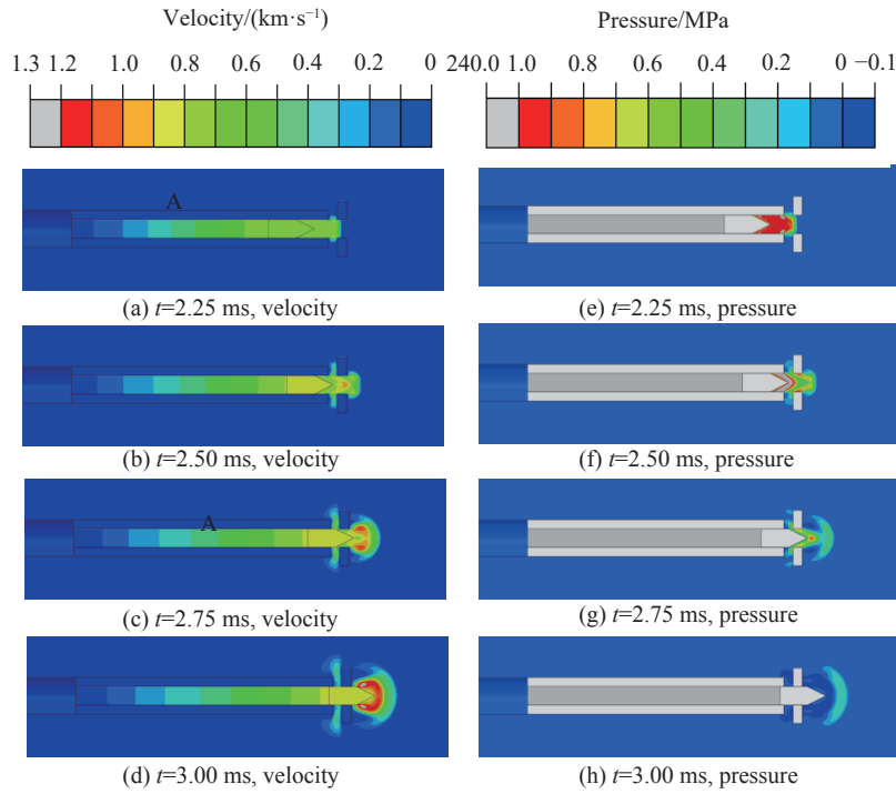
图 4 初始冲击波流场速度和流场压力的动态演化
