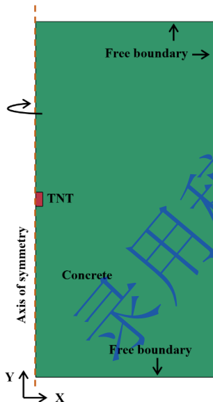
图 5 有限元模型
