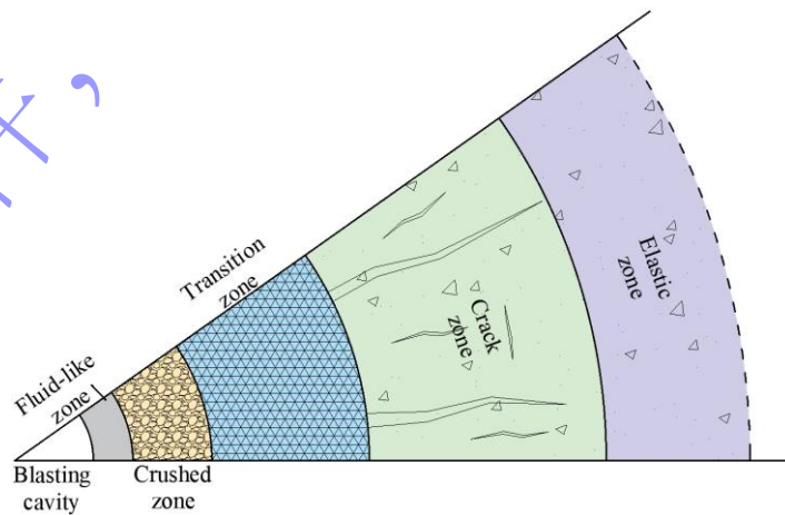
图 6 装药周围介质破坏分区
